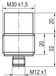
Габаритный чертеж
